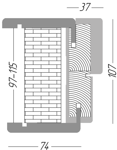
Телескопічний BRANDU з пласкою лиштвою
