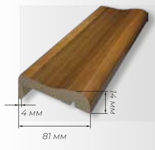
Лиштва «Хвиля», телескопічна
